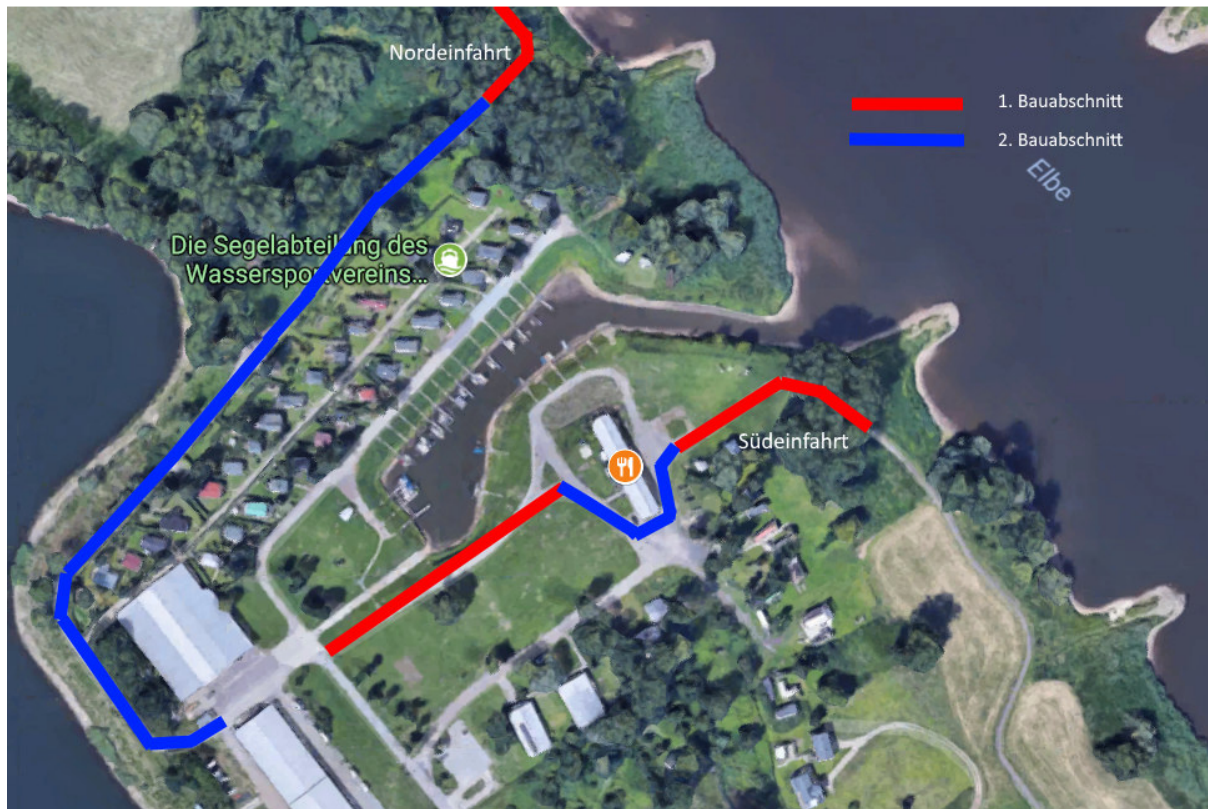
Übersicht Lage und Bauabschnitte
